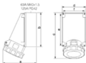
TOMADA 63A - 125A
